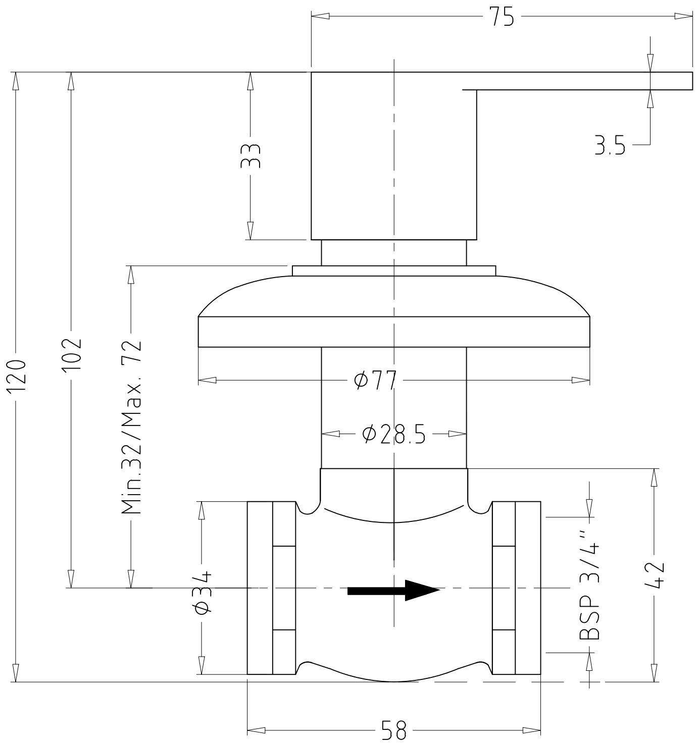
ASPIRO:F570008 CONCEALED STOP COCK 20 MM WITH FLANGE
