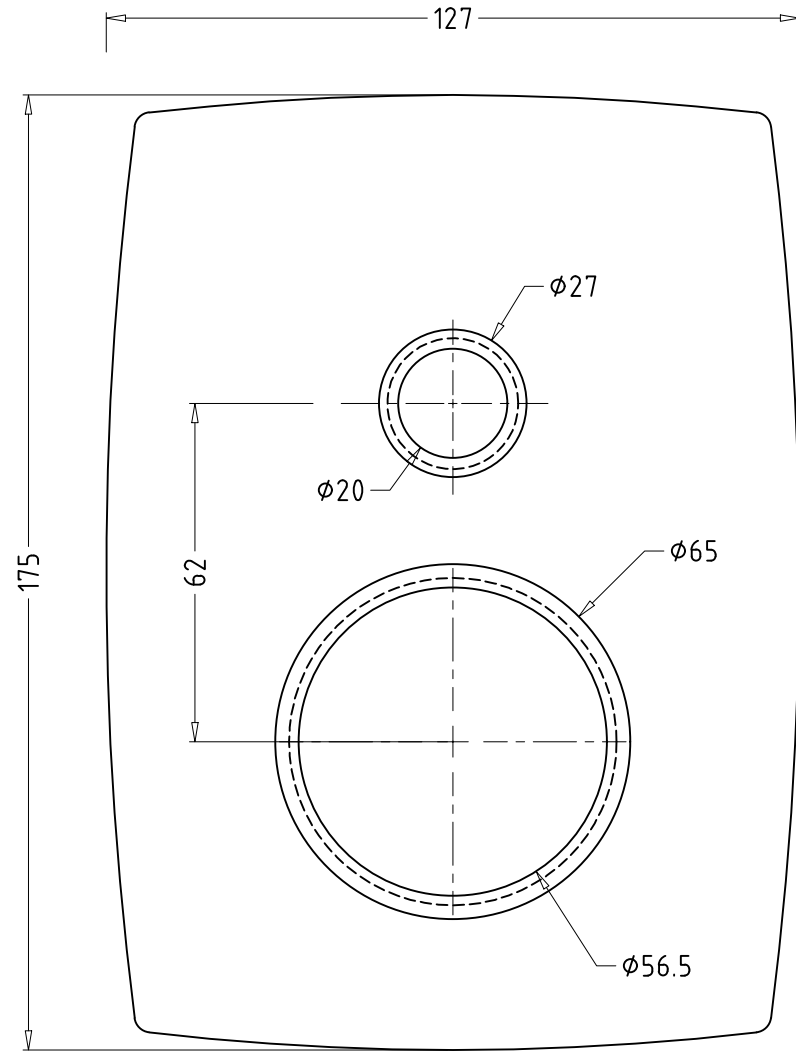
ASPIRO : 3 INLET PLATE
